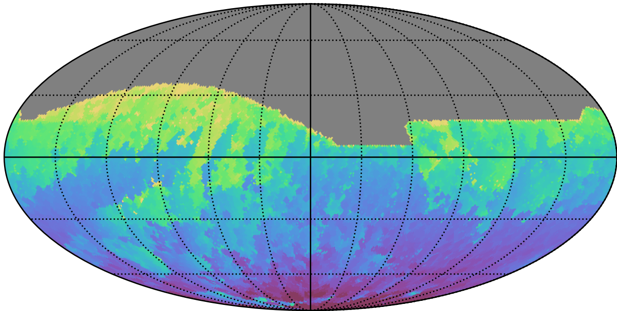
ddf_acor_sf10_lsf40_lsr50_v3.4_10yrs All sky z band: Min HA
