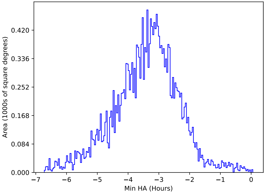
ddf_acor_sf10_lsf40_lsr50_v3.4_10yrs All sky y band: Min HA
