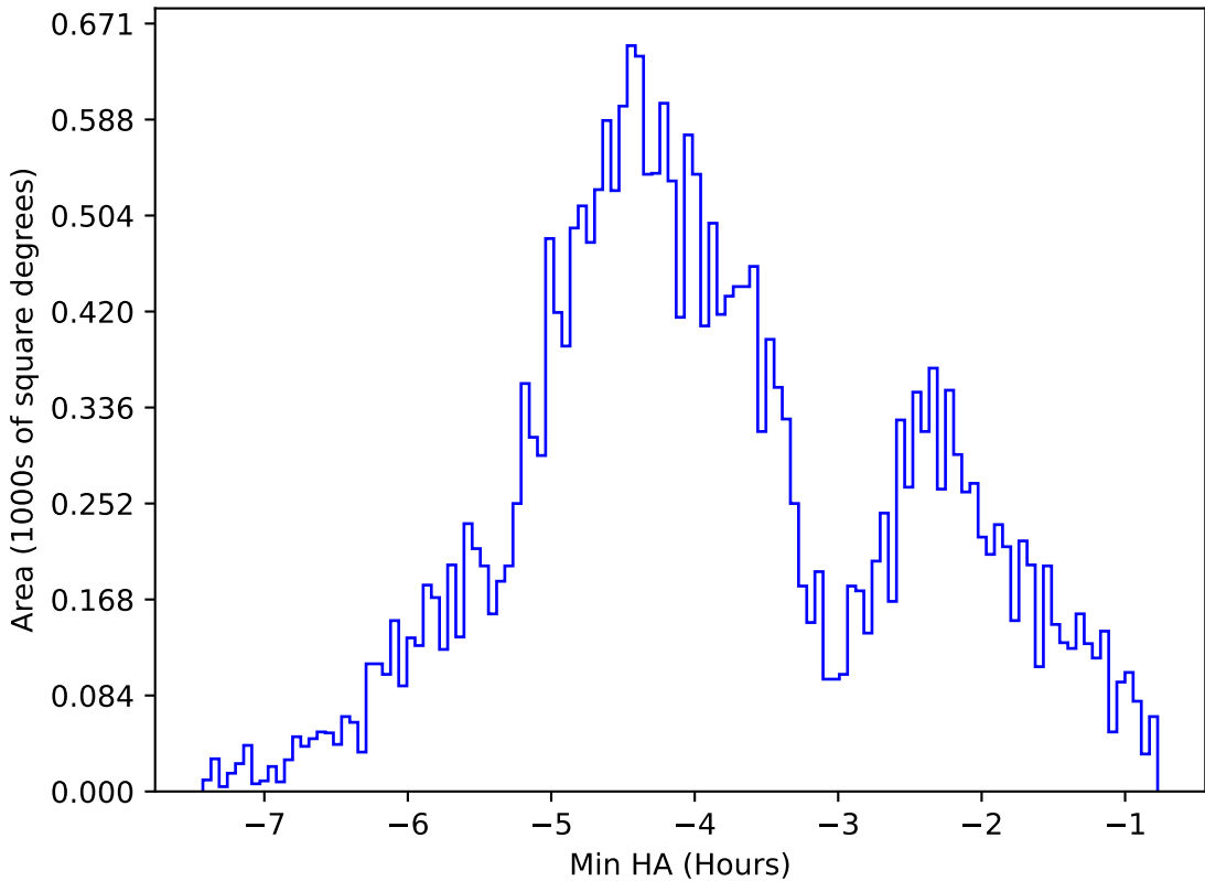
ddf_acor_sf10_lsf40_lsr50_v3.4_10yrs All sky g band: Min HA
