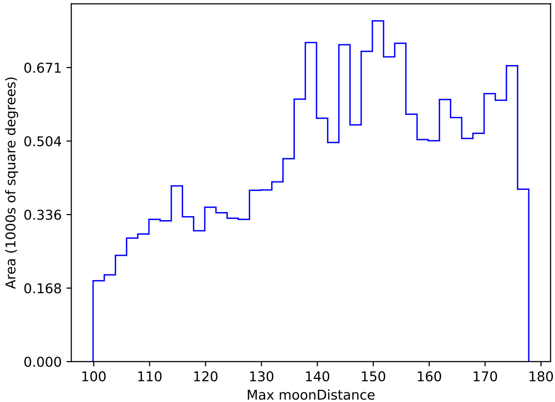
ddf_acor_sf10_lsf40_lsr50_v3.4_10yrs WFD y band: Max moonDistance
