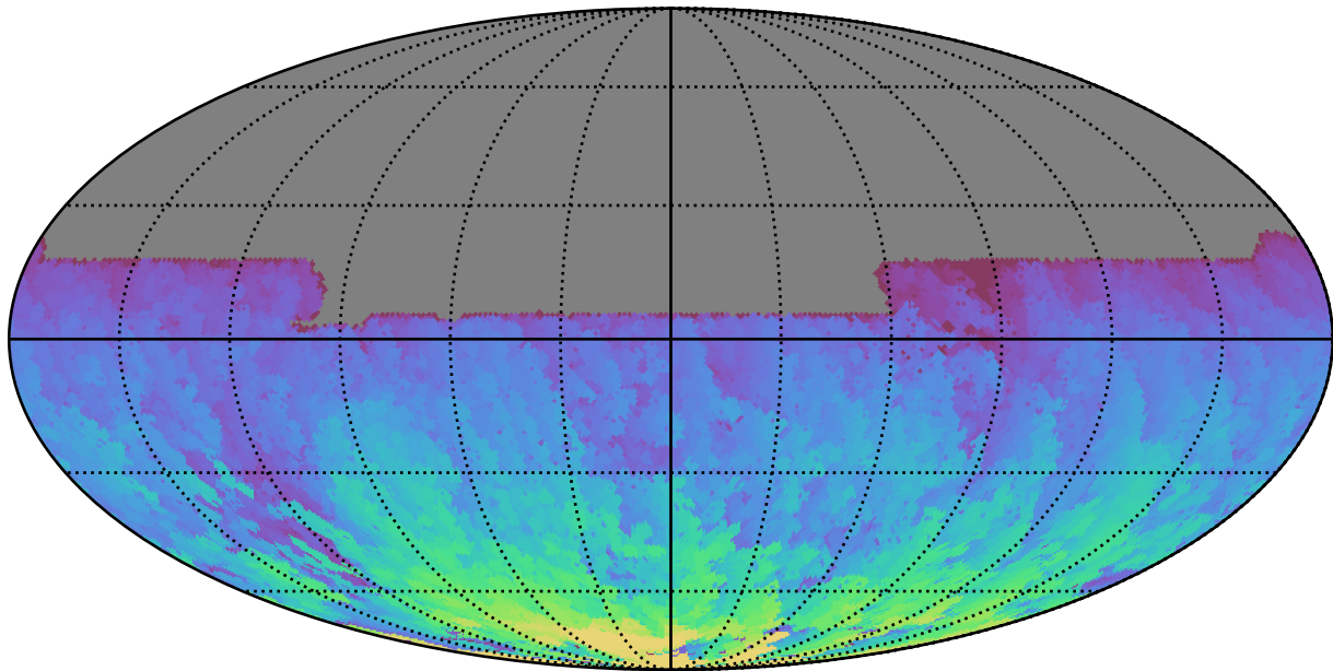
ddf_acor_sf10_lsf40_lsr50_v3.4_10yrs All sky y band: Max HA
