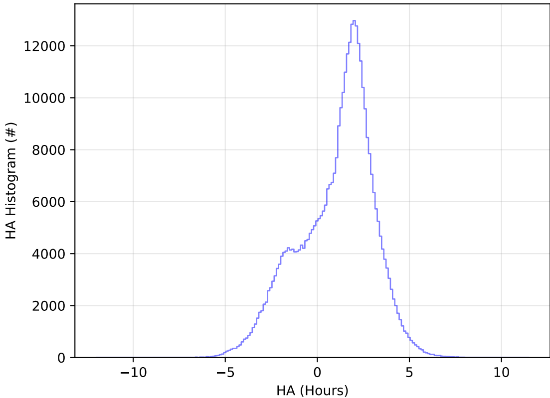
ddf_acor_sf10_lsf40_lsr50_v3.4_10yrs All sky y band: HA Histogram
