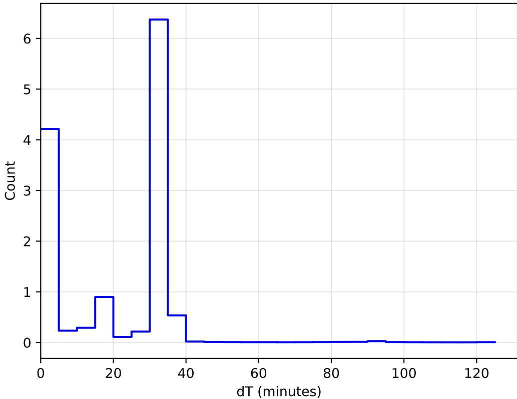
ddf_acor_sf10_lsf40_lsr50_v3.4_10yrs All sky: DeltaT Histogram
