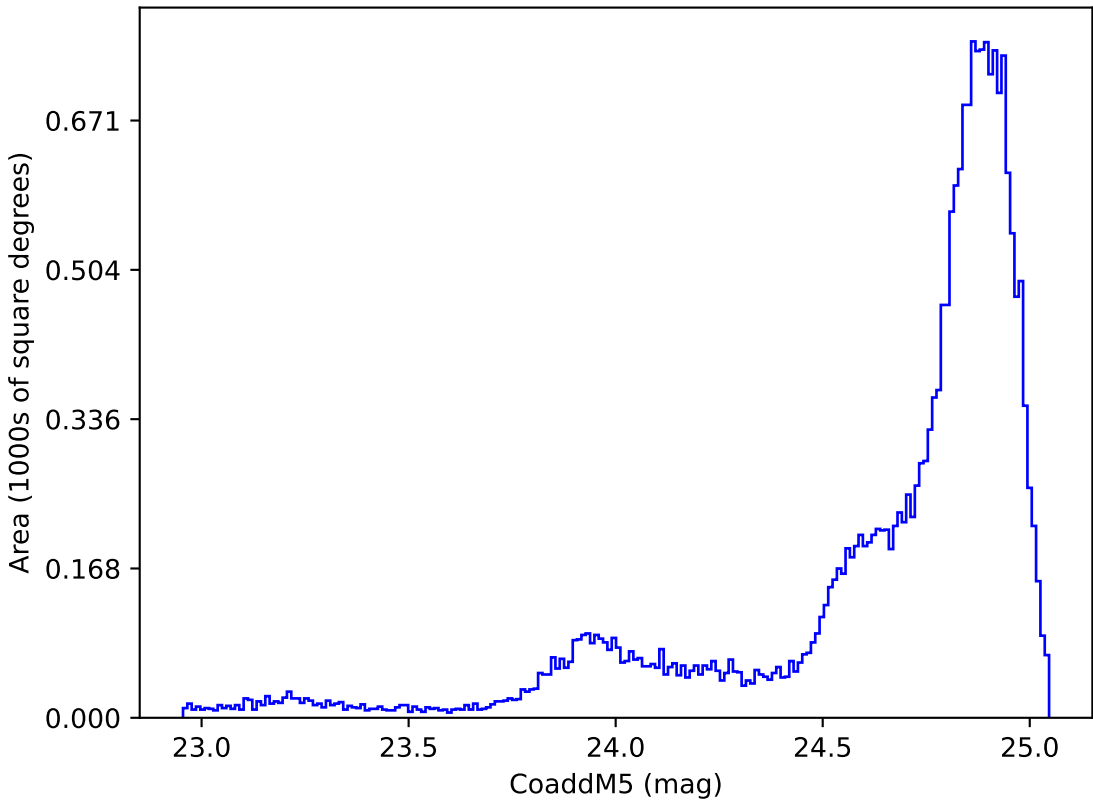
ddf_acor_sf10_lsf40_lsr50_v3.4_10yrs All sky y band: CoaddM5
