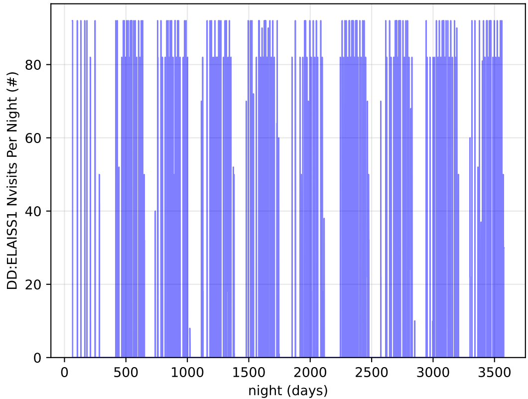
ddf_acor_sf10_lsf40_lsr50_v3.4_10yrs all bands: DD:ELAISS1 Nvisits Per Night
