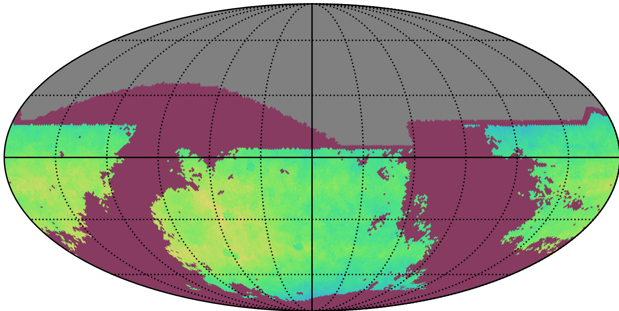
ddf_acor_sf10_lsf40_lsr20_v3.4_10yrs i: NgalScale
