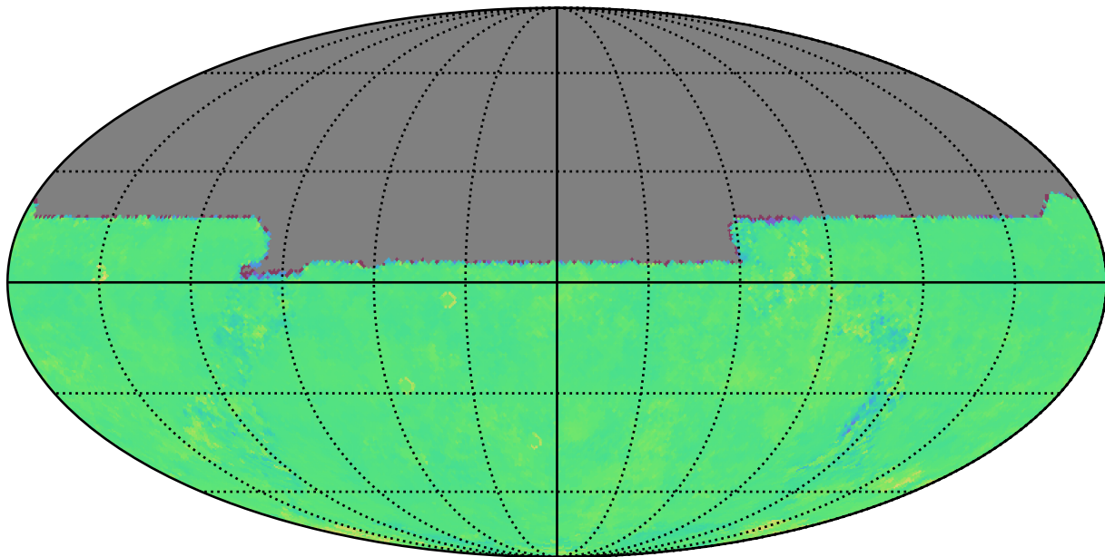
ddf_acor_sf10_lsf40_lsr20_v3.4_10yrs u: Kuiper rotTelPos
