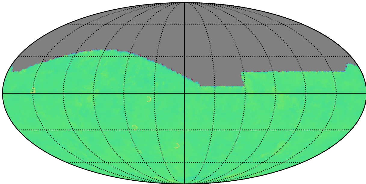
ddf_acor_sf10_lsf40_lsr20_v3.4_10yrs i: Kuiper rotTelPos
