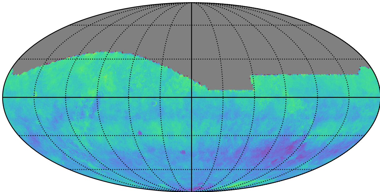
ddf_acor_sf10_lsf40_lsr20_v3.4_10yrs i: Kuiper rotSkyPos
