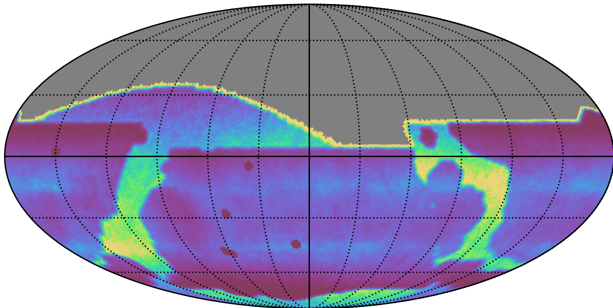
ddf_acor_sf10_lsf40_lsr20_v3.4_10yrs : DCRprecision
