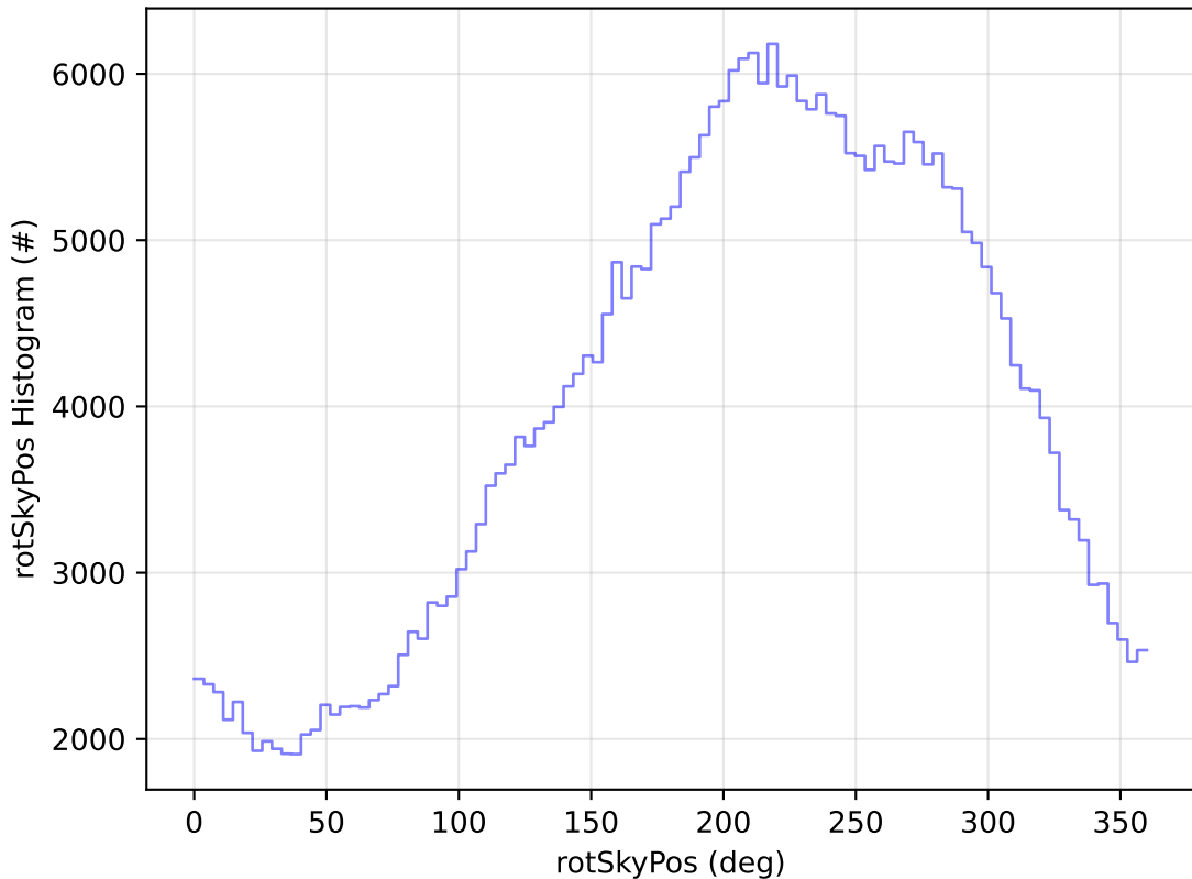
ddf_acor_sf10_lsf40_lsr20_v3.4_10yrs All sky y band: rotSkyPos Histogram
