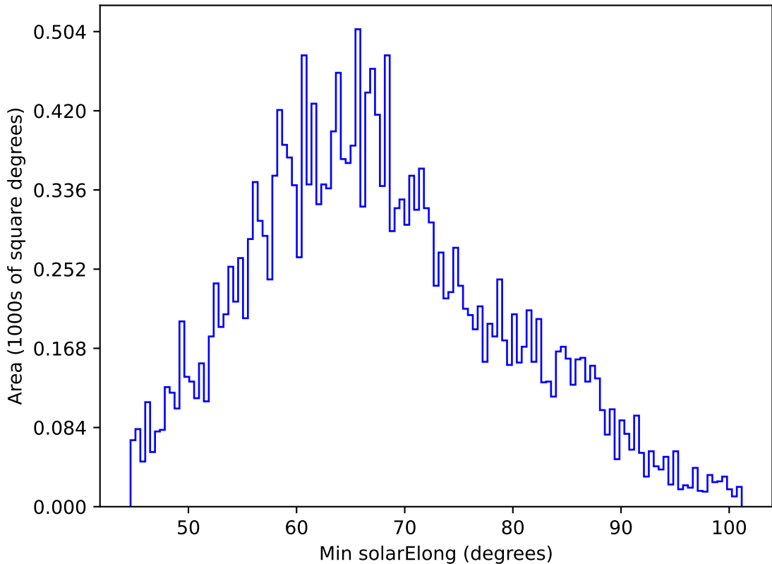
ddf_acor_sf10_lsf40_lsr20_v3.4_10yrs All sky y band: Min solarElong
