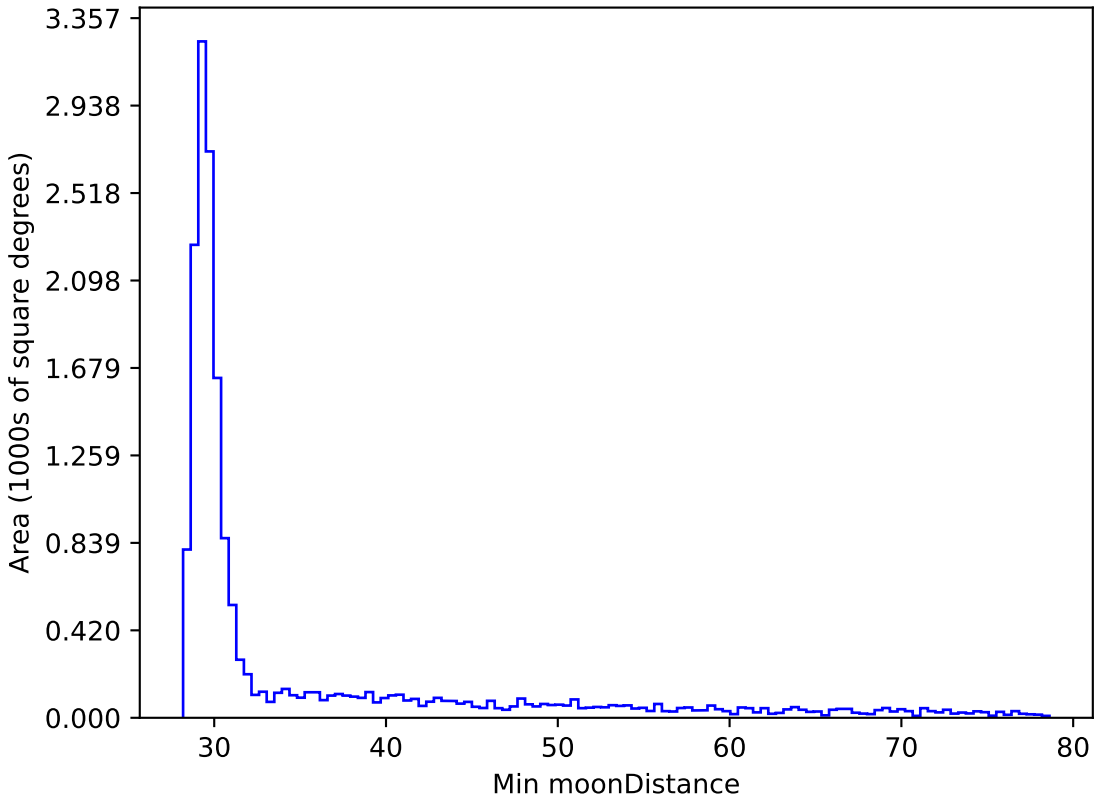
ddf_acor_sf10_lsf40_lsr20_v3.4_10yrs WFD y band: Min moonDistance
