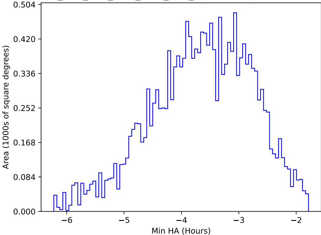
ddf_acor_sf10_lsf40_lsr20_v3.4_10yrs WFD y band: Min HA
