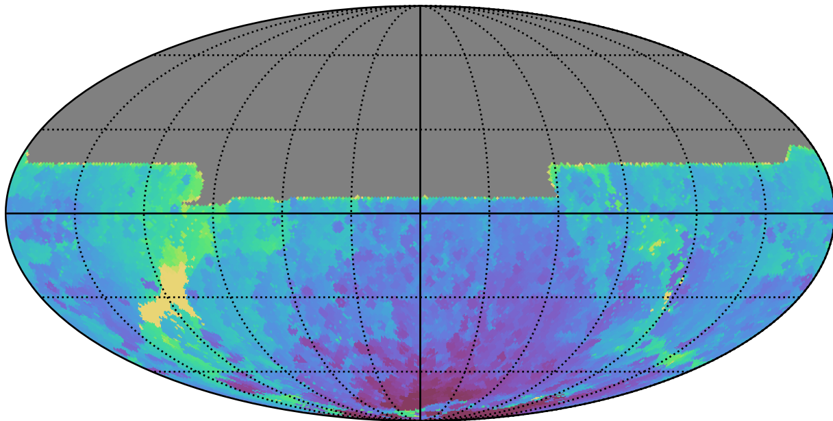
ddf_acor_sf10_lsf40_lsr20_v3.4_10yrs All sky y band: Min HA
