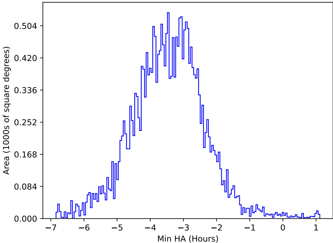
ddf_acor_sf10_ls40_lsr20_v3.4_10yrs All sky y band: Min HA
