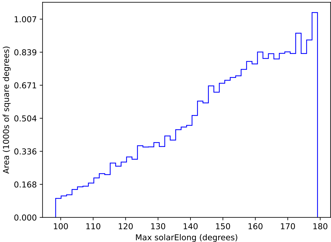
ddf_acor_sf10_lsf40_lsr20_v3.4_10yrs All sky y band: Max solarElong
