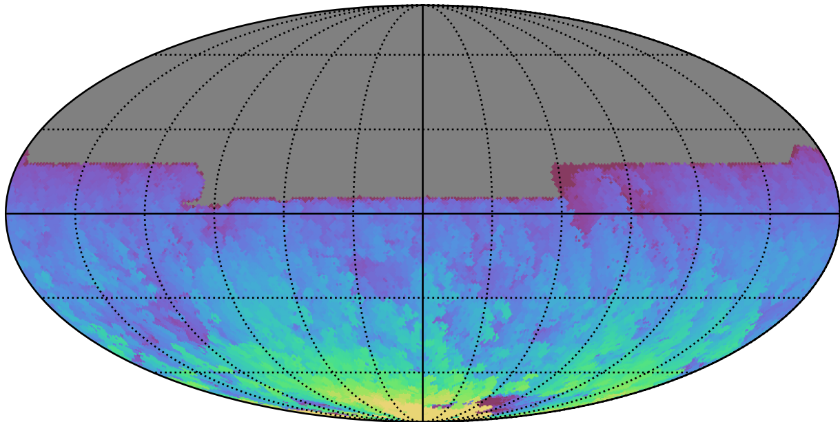
ddf_acor_sf10_lsf40_lsr20_v3.4_10yrs All sky y band: Max HA
