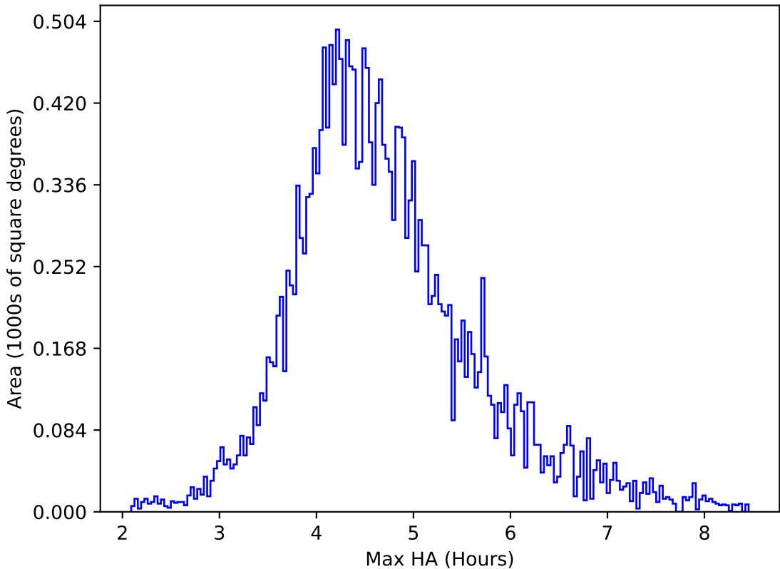
ddf_acor_sf10_lsf40_lsr20_v3.4_10yrs All sky y band: Max HA
