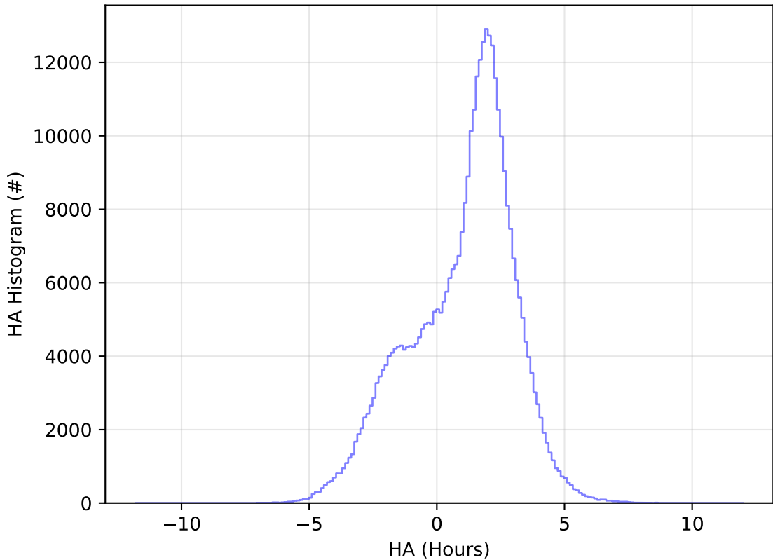
ddf_acor_sf10_lsf40_lsr20_v3.4_10yrs All sky y band: HA Histogram
