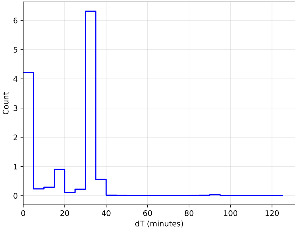
ddf_acor_sf10_lsf40_lsr20_v3.4_10yrs All sky: DeltaT Histogram
