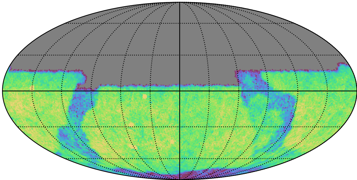
ddf_acor_sf10_lsf40_lsr20_v3.4_10yrs Yr 1 y band: CoaddM5
