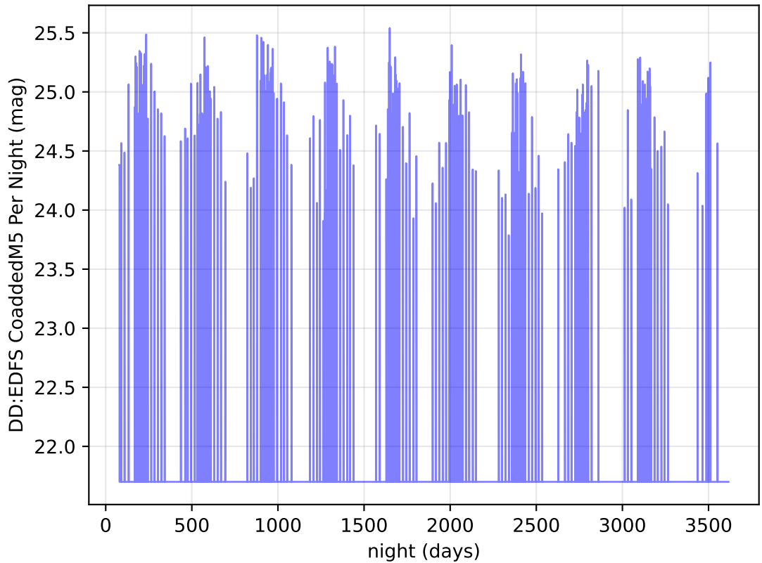
ddf_acor_sf10_lsf40_lsr20_v3.4_10yrs z band: DD:EDFS CoaddedM5 Per Night
