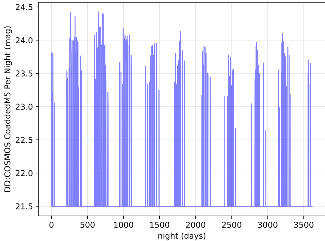
ddf_acor_sf10_lsf40_lsr20_v3.4_10yrs y band: DD:COSMOS CoaddedM5 Per Night
