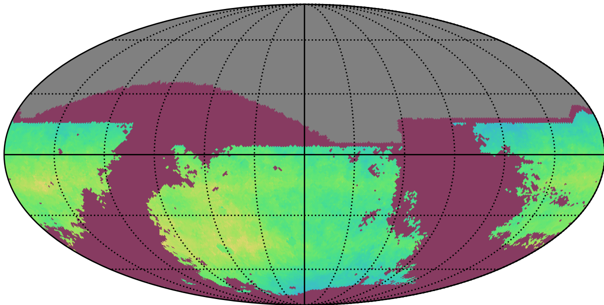
ddf_acor_sf10_lsf40_lsr10_v3.4_10yrs i: NgalScale
