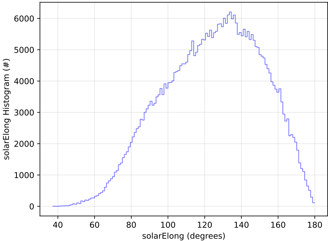
ddf_acor_sf10_lsf40_lsr10_v3.4_10yrs All sky y band: solarElong Histogram
