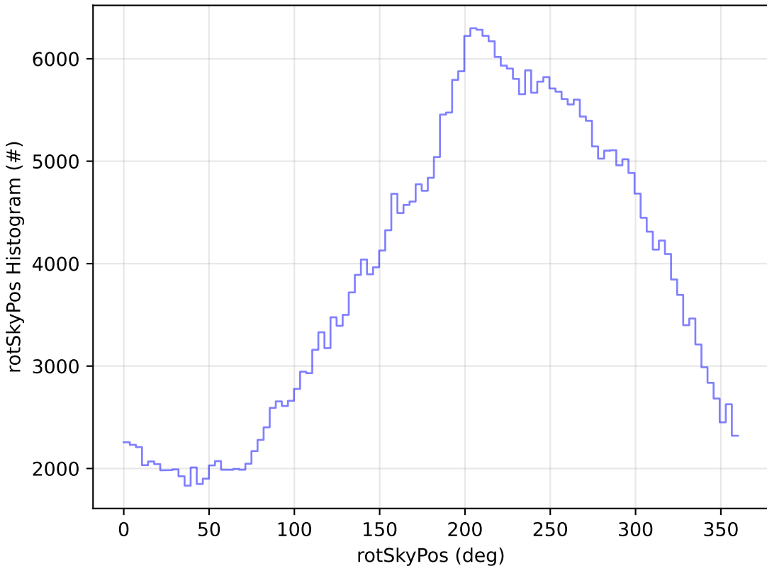
ddf_acor_sf10_lsf40_lsr10_v3.4_10yrs All sky y band: rotSkyPos Histogram
