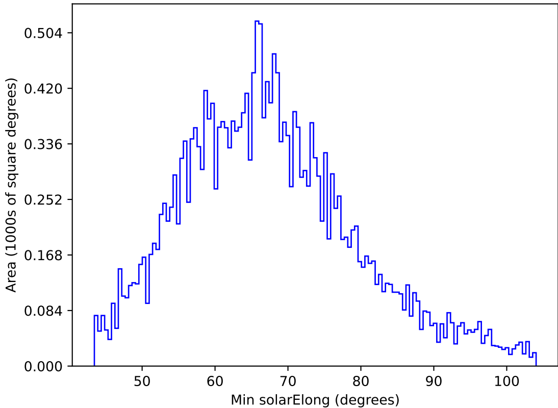
ddf_acor_sf10_lsf40_lsr10_v3.4_10yrs All sky y band: Min solarElong
