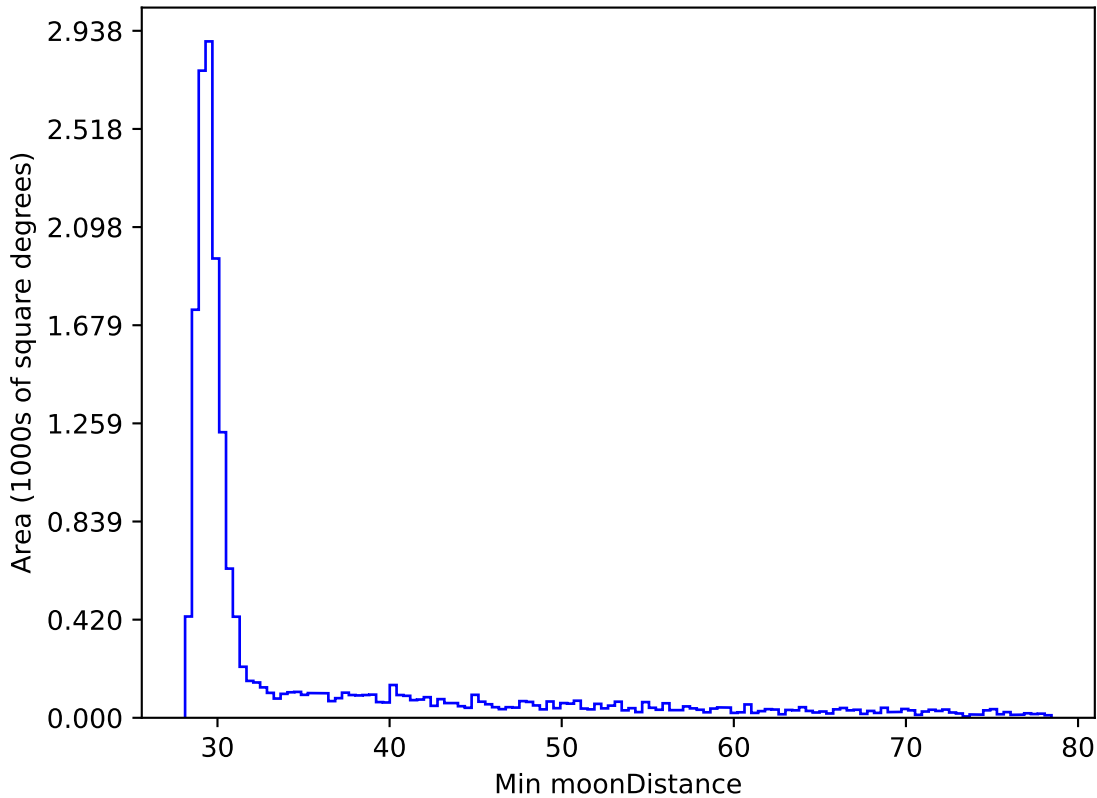
ddf_acor_sf10_lsf40_lsr10_v3.4_10yrs WFD y band: Min moonDistance
