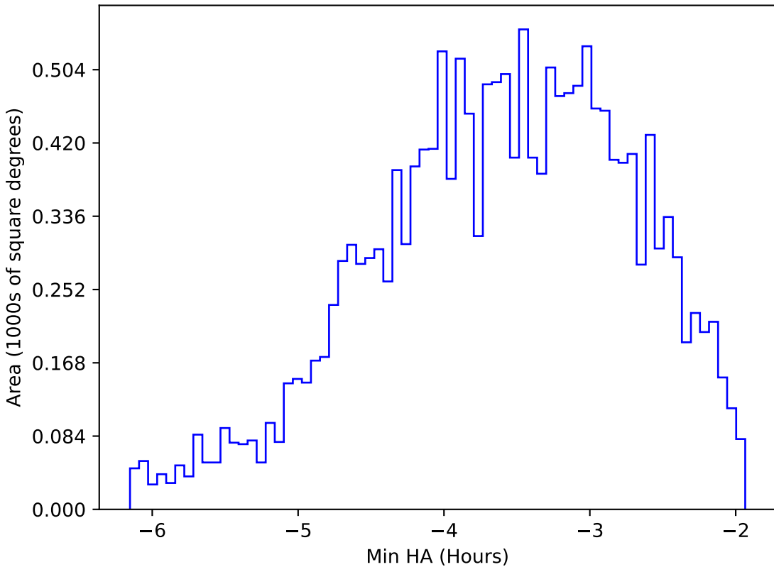
ddf_acor_sf10_lsf40_lsr10_v3.4_10yrs WFD y band: Min HA
