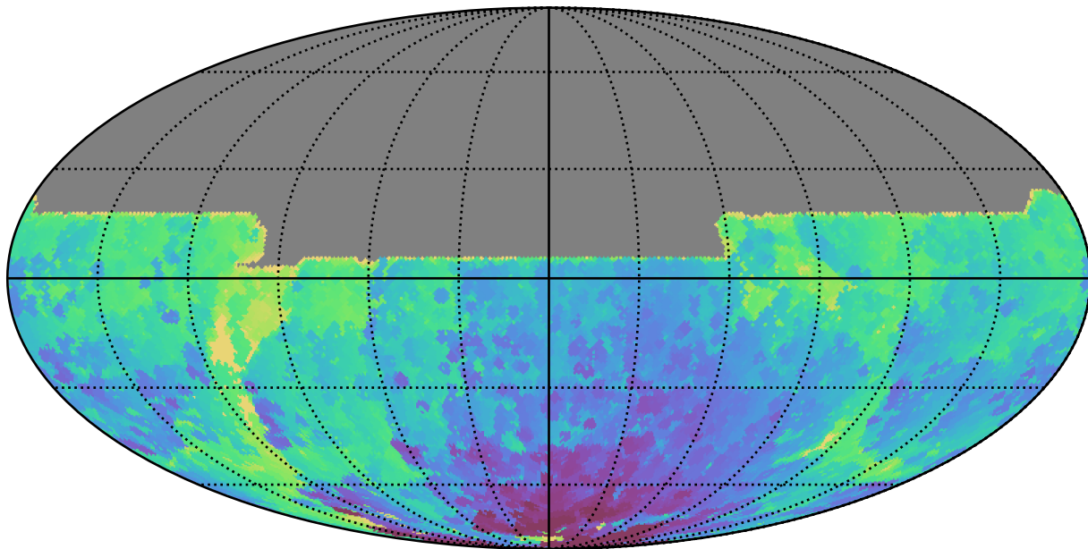
ddf_acor_sf10_lsf40_lsr10_v3.4_10yrs All sky y band: Min HA
