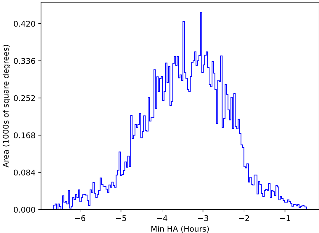
ddf_acor_sf10_lsf40_lsr10_v3.4_10yrs All sky y band: Min HA
