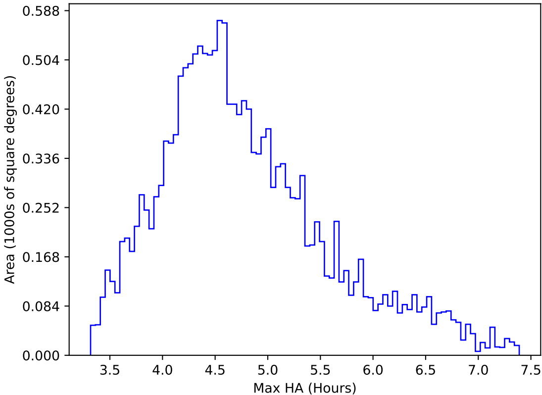
ddf_acor_sf10_lsf40_lsr10_v3.4_10yrs WFD y band: Max HA
