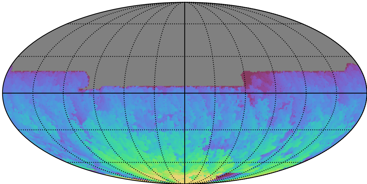
ddf_acor_sf10_lsf40_lsr10_v3.4_10yrs All sky y band: Max HA
