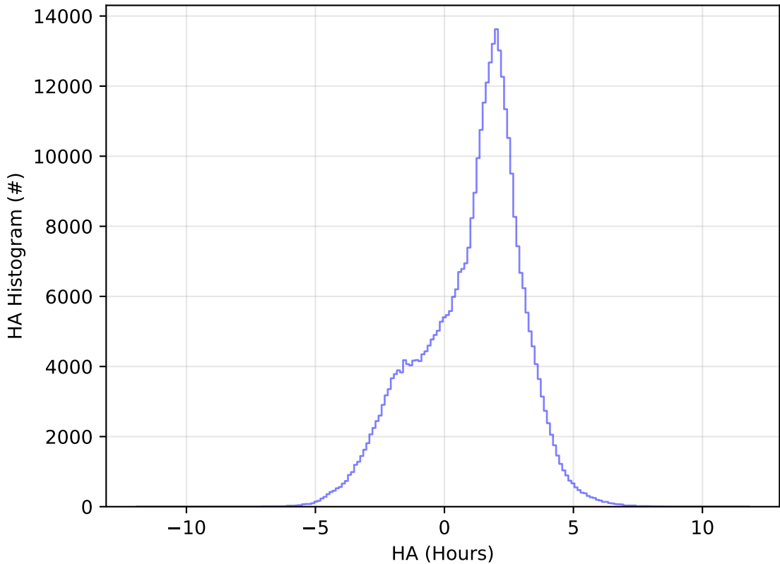
ddf_acor_sf10_lsf40_lsr10_v3.4_10yrs All sky y band: HA Histogram
