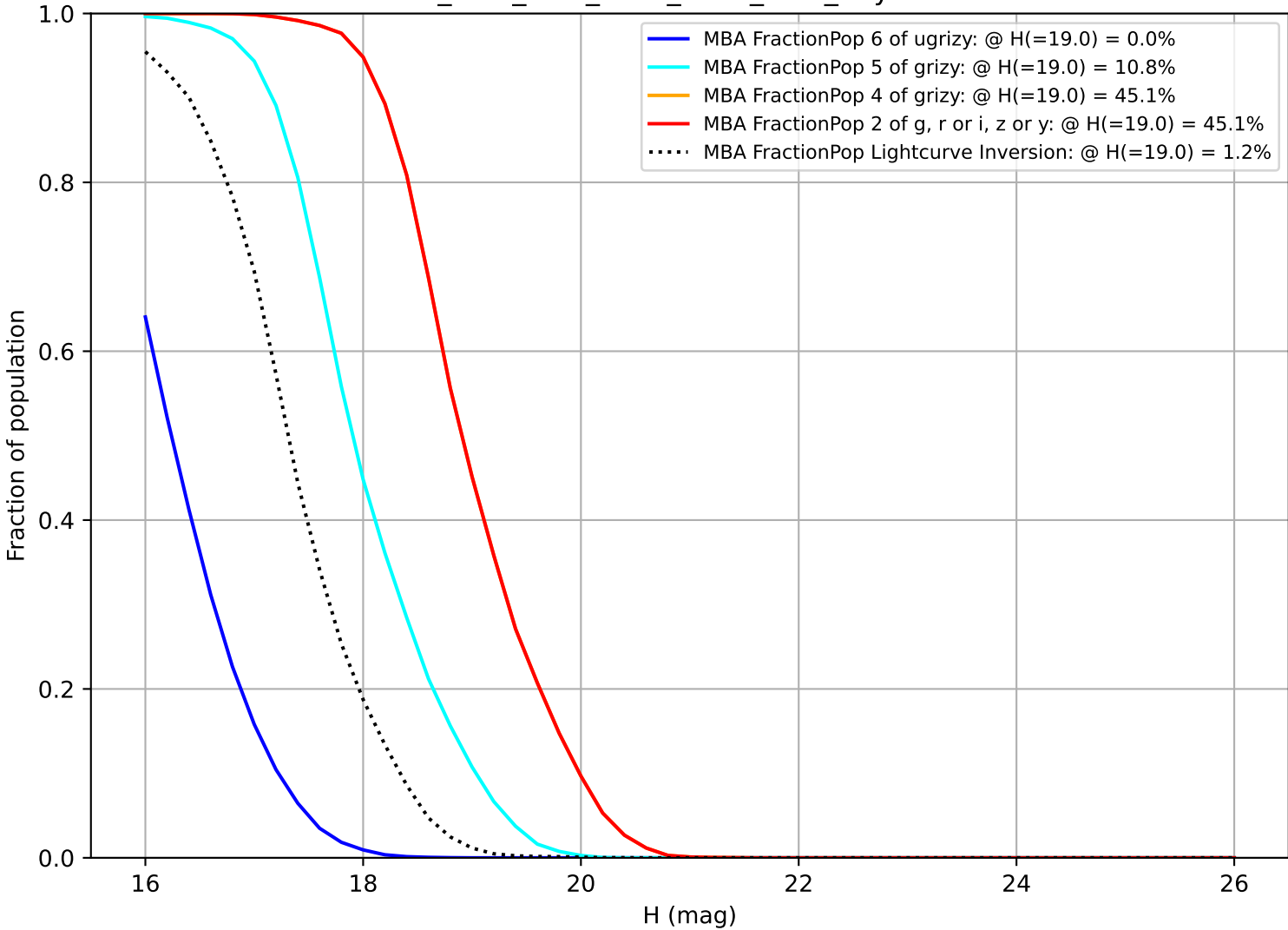
ddf_acor_sf10_lsf30_lsr50_v3.4_10yrs MBA
