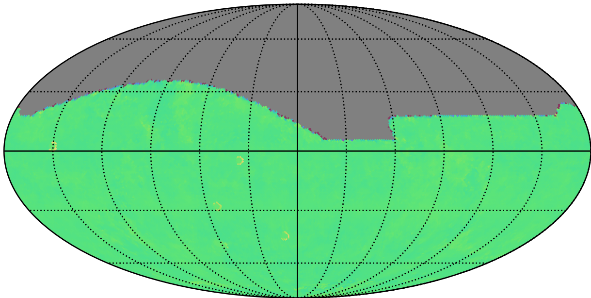
ddf_acor_sf10_lsf30_lsr50_v3.4_10yrs i: Kuiper rotTelPos
