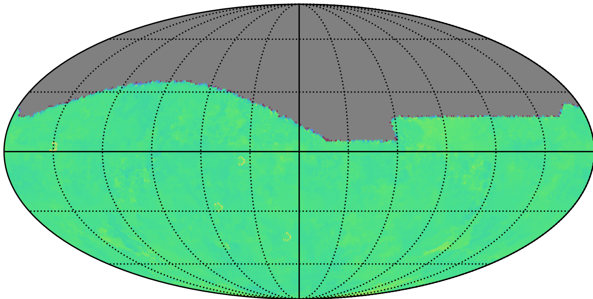
ddf_acor_sf10_lsf30_lsr50_v3.4_10yrs g: Kuiper rotTelPos
