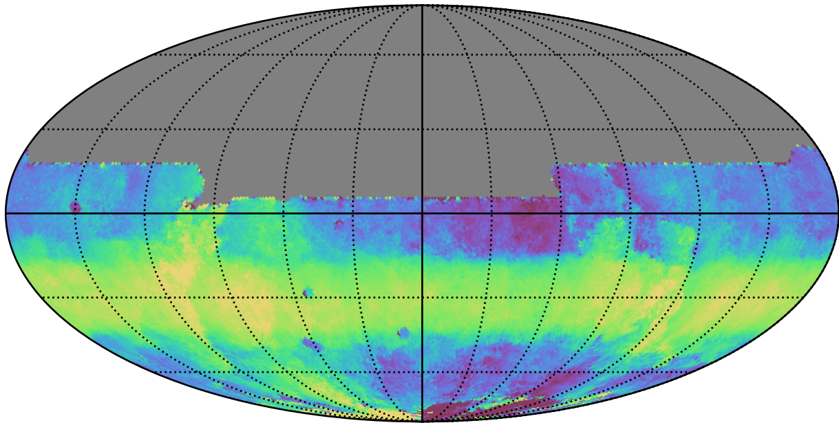
ddf_acor_sf10_lsf30_lsr50_v3.4_10yrs All sky y band: Median HA
