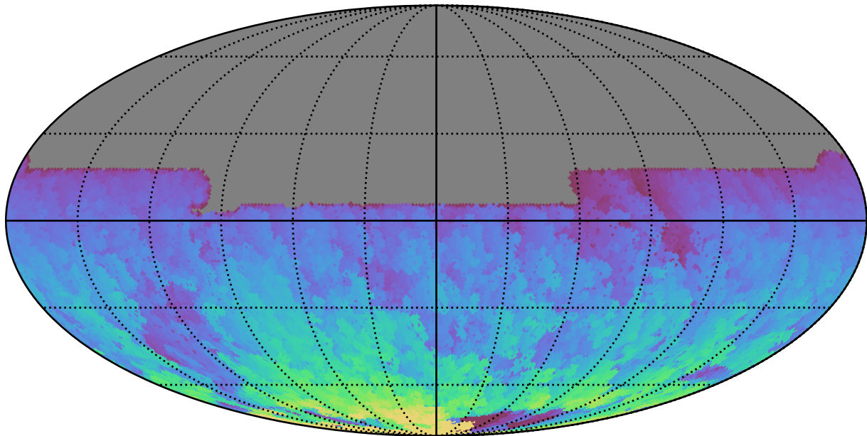
ddf_acor_sf10_lsf30_lsr50_v3.4_10yrs All sky y band: Max HA
