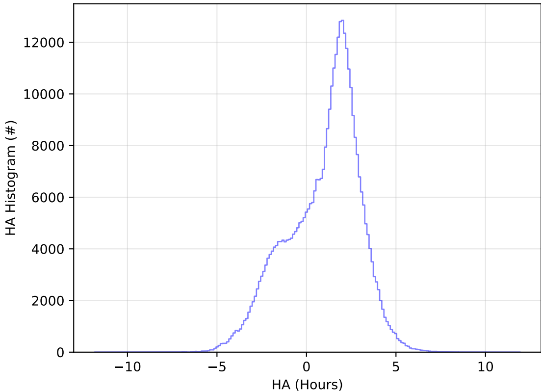
ddf_acor_sf10_lsf30_lsr50_v3.4_10yrs All sky y band: HA Histogram
