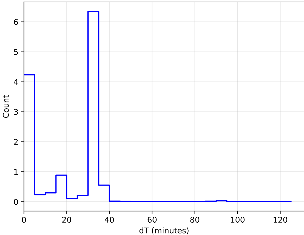
ddf_acor_sf10_lsf30_lsr50_v3.4_10yrs All sky: DeltaT Histogram
