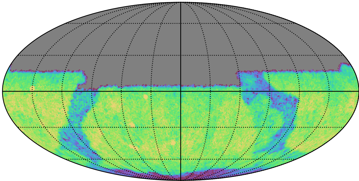
ddf_acor_sf10_lsf30_lsr50_v3.4_10yrs Yr 1 y band: CoaddM5
