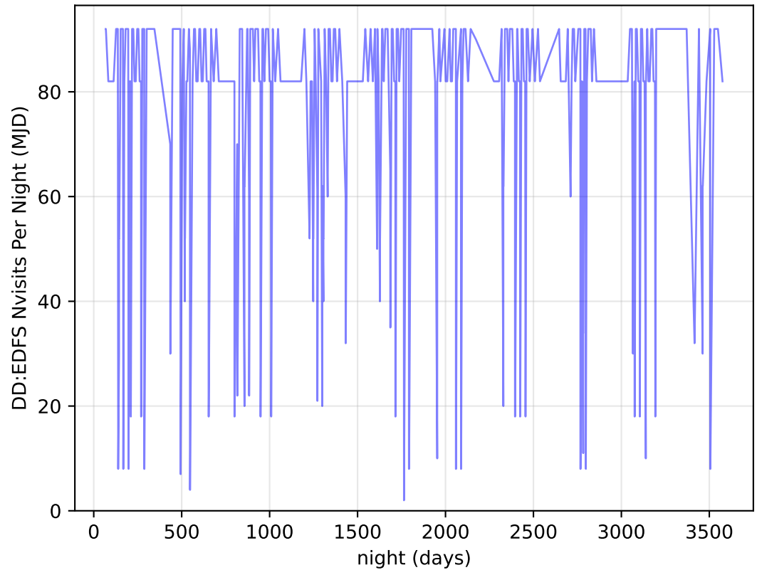
ddf_acor_sf10_lsf30_lsr50_v3.4_10yrs all bands: DD:EDFS Nvisits Per Night
