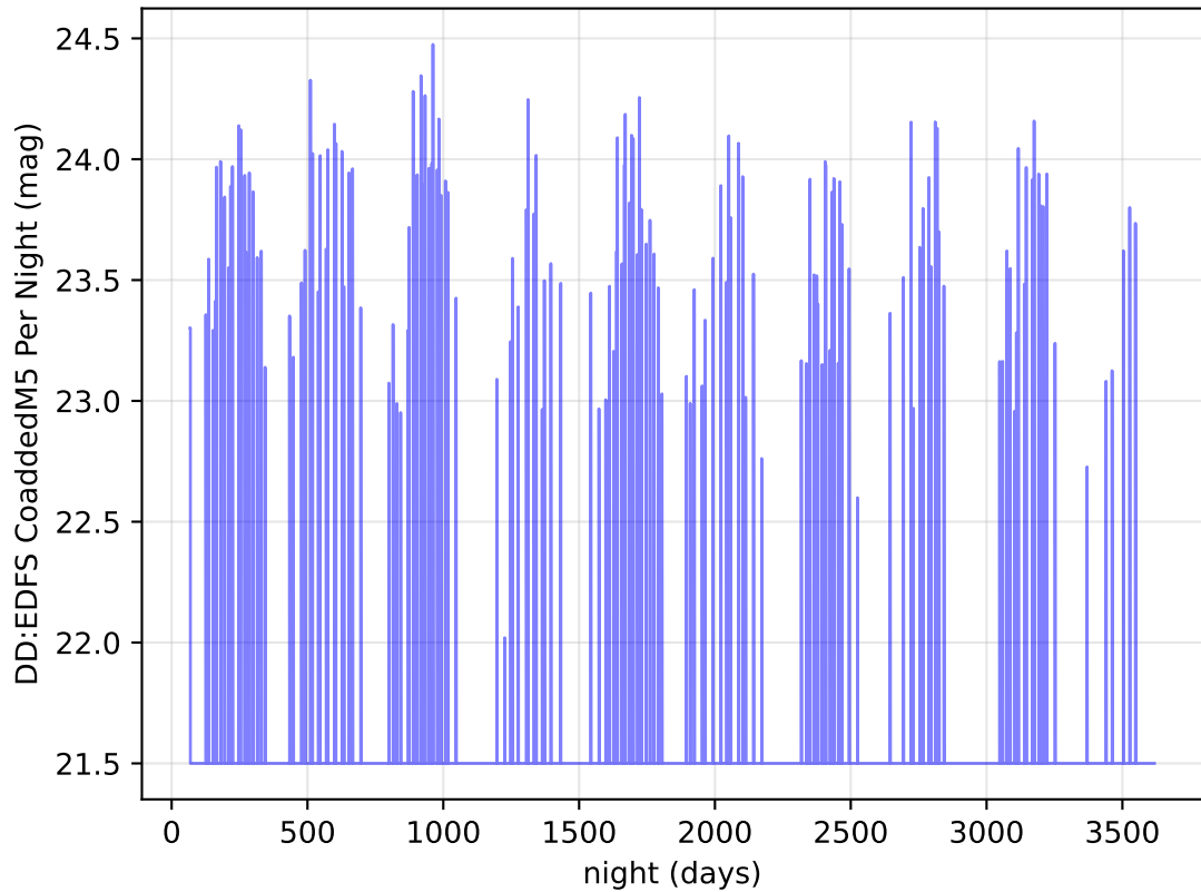
ddf_acor_sf10_lsf30_lsr50_v3.4_10yrs y band: DD:EDFS CoaddedM5 Per Night
