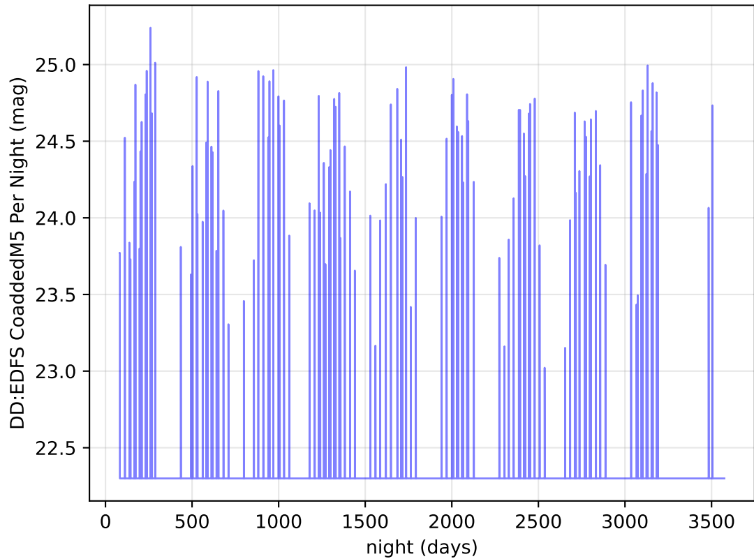
ddf_acor_sf10_lsf30_lsr50_v3.4_10yrs u band: DD:EDFS CoaddedM5 Per Night
